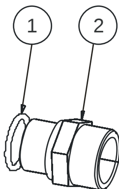
1S02K260 (No. 12) Adaptador XAL 15 3/4" – 16 UNF
